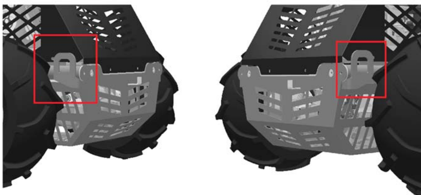
Puntos de anclaje para cuerdas o bandas para "bloquear" la máquina en furgonetas o camiones
